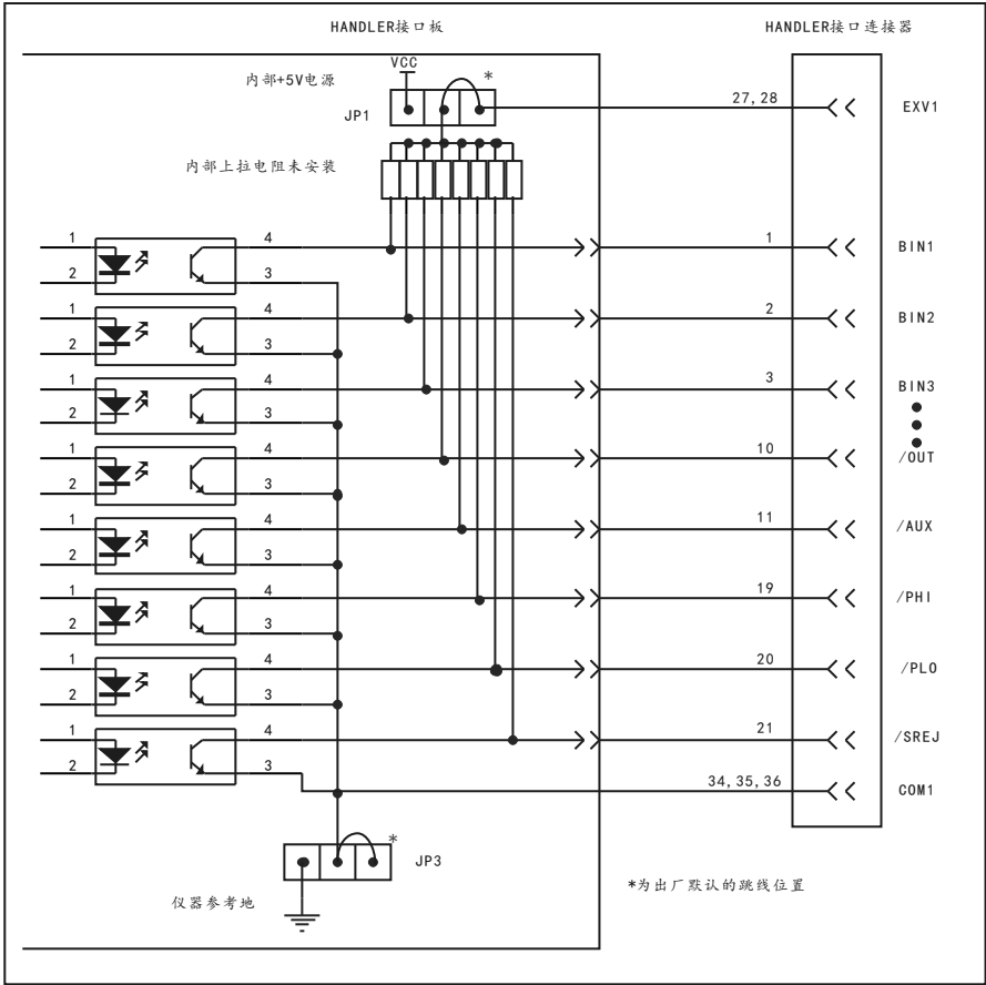
分选输出信号电气示意图：
