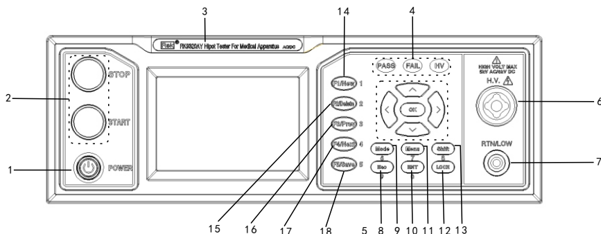
图 3-1 前面板说明
