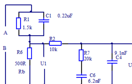
MD-C (兼容IEC60990图5的U3测试)
