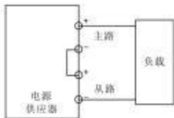
单电源串联模式
